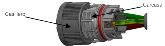
Figura 4.16 Conectar los cables al terminal
