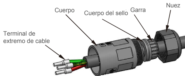
Figura 4.14 Conector de terminal de red de CA
