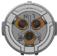
Figura 4.13 Conector de terminal de red de CA en el interior
